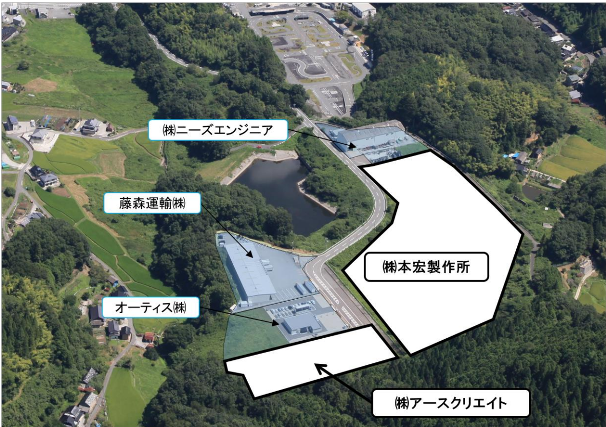
新見工業団地平面図
